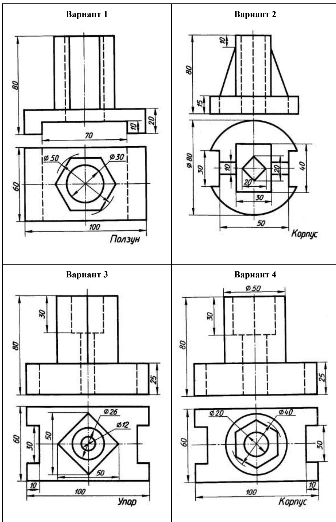
Рисунок 3.11 – Разрезы простые
